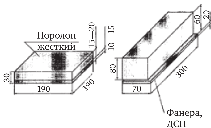
Рис. 10.4. Подлокотник и валик
