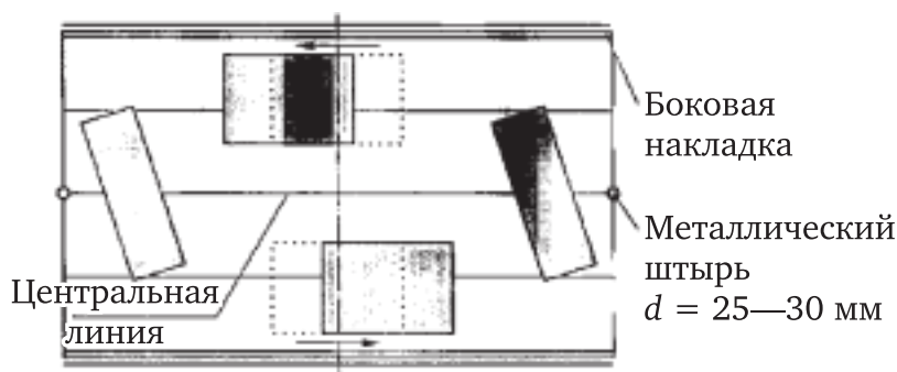
Рис. 10.3. Щит армстола для борьбы правой рукой с разнесенными подлокотниками (вид сверху)
