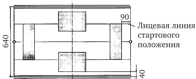
Рис. 10.2. Щит армстола (вид сверху)
