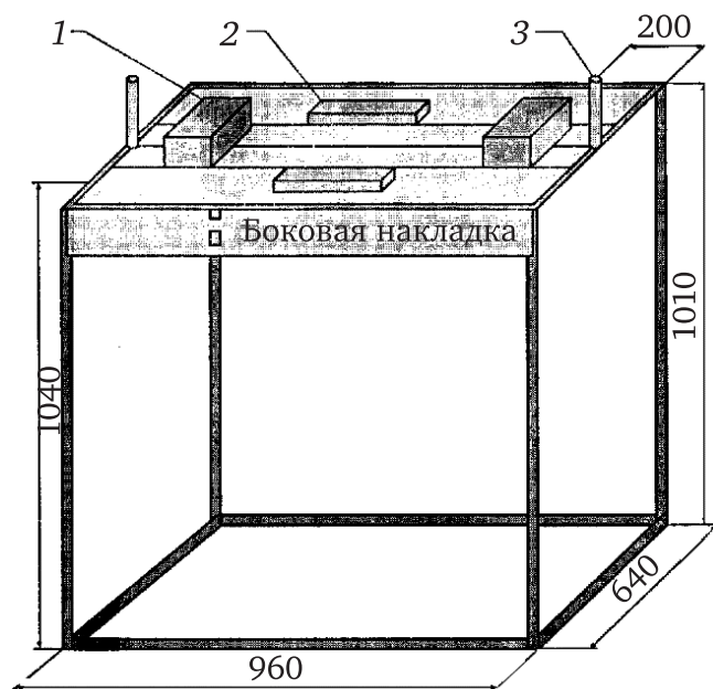
Рис. 10.1. Общий вид армстола:
