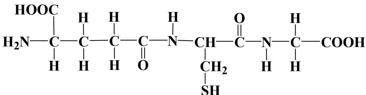
Рис.8. α- и γ-пептидные связи
