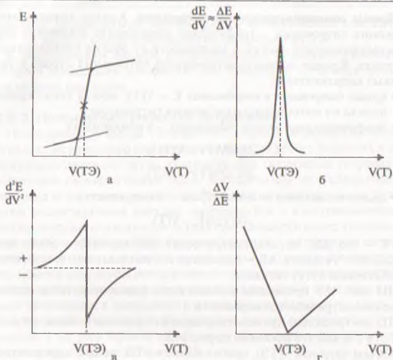
Рис. 17.3. Типы кривых потенциометрического титрования ( E — измеряемая ЭДС, V(T) — объем прибавленного титранта, V(TЭ) — объем титранта, прибавленного в точке эквивалентности): a — кривая в координатах E - V(T) ; б, в — дифференциальные кривые титрования; г — кривая титрования по методу Грана.
