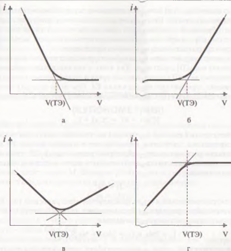
Рис. 23.5. Типы кривых амперометрического титрования:
