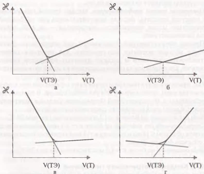
Рис. 15.8. Схематическое изображение некоторых типов кривых кондуктометрического титрования ( \kappa — удельная электропроводность; V(T) — объем прибавленного титранта): а — титрование раствора сильной кислоты раствором щелочи; б — титруемое вещество и титрант имеют ионы с низкой электрической подвижностью; в — титрование сильной кислоты раствором гидрокарбоната натрия; г — титруемое вещество имеет ионы с малой электрической подвижностью, титрант — с более высокой электрической подвижностью.
