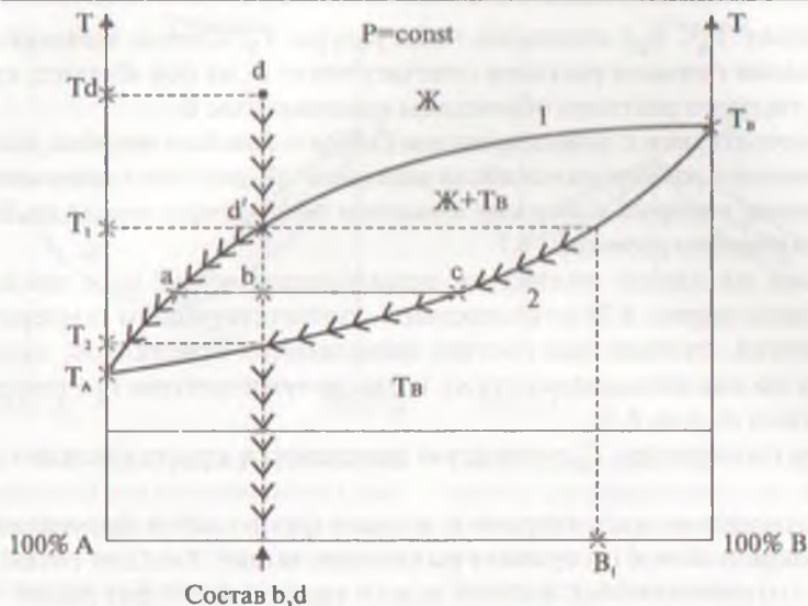
Рис. 8.3. Диаграмма состояния (плавкости) бинарной системы из двух компонентов А и В, неограниченно растворимых друг в друге.
