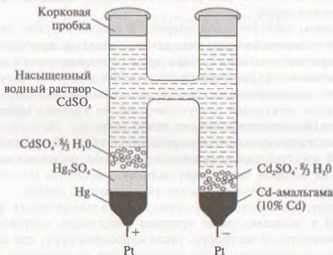
Рис. 17.1. Схема насыщенного элемента Вестона (простая химическая цепь).
