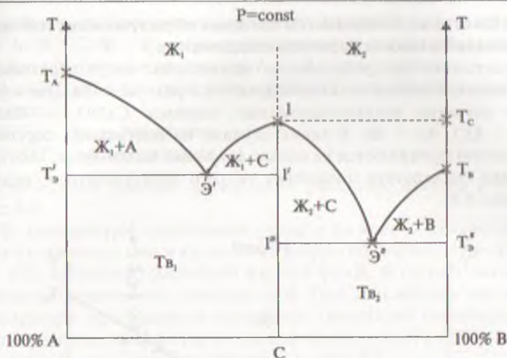
Рис. 8.7. Диаграмма состояния (плавкости) двухкомпонентной системы, в которой компоненты А и В образуют одно плавящееся конгруэнтно соединение С.
