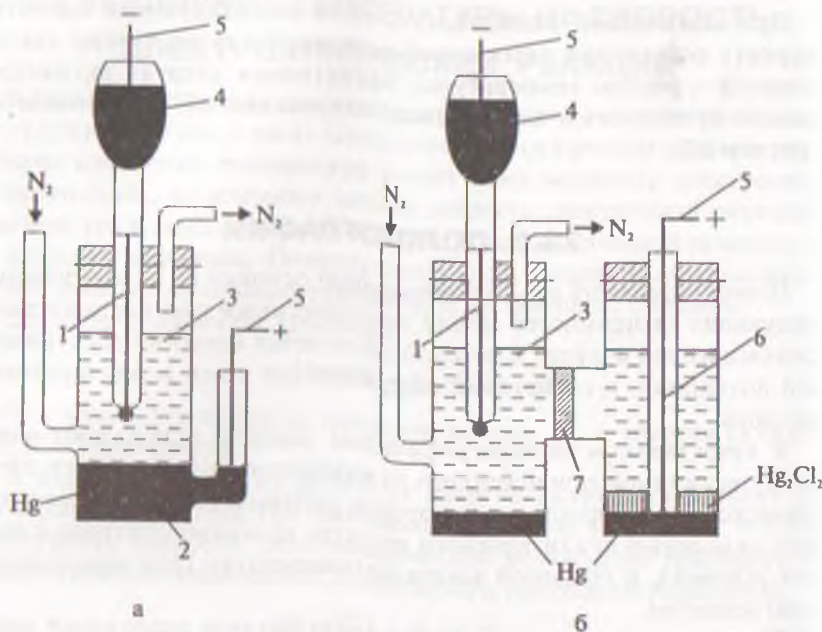
Рис. 23.2. Схема полярографической ячейки с ртутным каплющим электродом и с ртутным анодом (а) или с насыщенным каломельным электродом (б): 1 — ртутный каплющий электрод, 2 — ртутный анод, 3 — анализируемый раствор, 4 — резервуар с жидкой ртутью, 5 — проводники к внешнему источнику постоянного тока, 6 — насыщенный каломельный электрод, 7 — пробка из пористого стекла.
