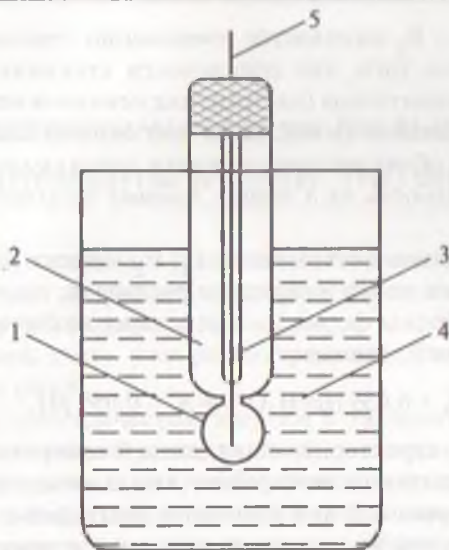
Рис. 16.2. Схема стеклянного электрода: 1 – стеклянный шарик (мембрана); 2 – внутренний раствор \text{HCl} ; 3 – хлорсеребряный электрод; 4 – измеряемый раствор; 5 – металлический проводник.
