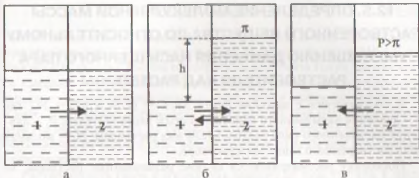
Рис. 12.3. Схема обратного осмоса: а — исходная система; б — осмотическое равновесие; в — обратный осмос. 1 — растворитель; 2 — раствор. Стрелками показано перемещение молекул растворителя через полупроницаемую мембрану. \pi — осмотическое давление, P — рабочее давление.
