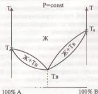
Рис. 8.4. Диаграмма состояния (плавкости) двухкомпонентной системы изоморфно кристаллизующихся компонентов А и В с минимумом температуры плавления.
