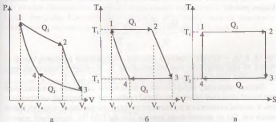
Рис. 3.1. Цикл Карно в координатах P - V (а), T - V (б), T - S (в): 1→2 — изотермическое расширение газа от объема V_1 до объема V_2 ; 2→3 — адиабатическое расширение газа от объема V_2 до объема V_3 ; 3→4 — изотермическое сжатие газа от объема V_3 до объема V_4 ; 4→1 — адиабатическое сжатие газа от объема V_4 до объема V_1 . Q_1 — теплота, поступающая из «нагревателя», Q_2 — теплота, возвращаемая «холодильнику» ( Q_2 < Q_1 ).
