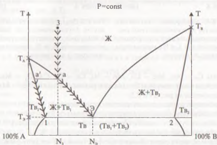
Рис. 8.6. Диаграмма состояния (плавкости) двухкомпонентной системы с неограниченной взаимной растворимостью компонентов А и В в жидком состоянии (расплав) и с ограниченной взаимной растворимостью компонентов в твердом состоянии, не образующих химических соединений.
