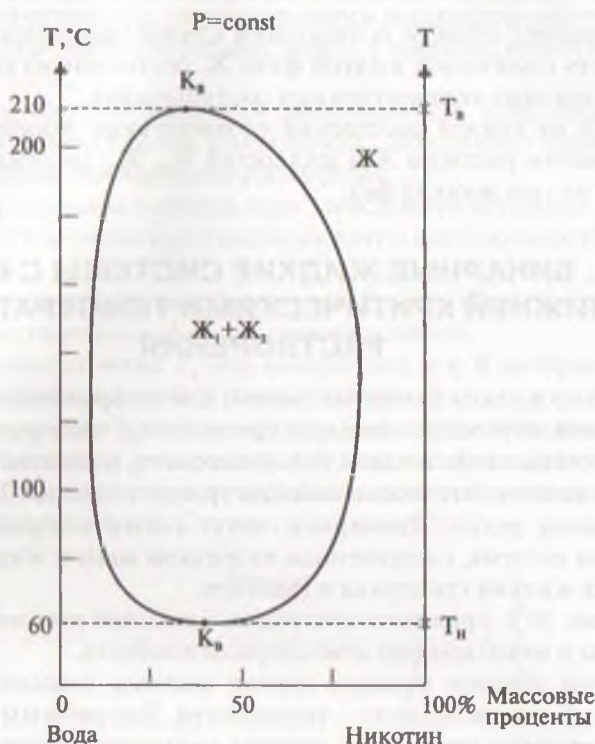
Рис. 10.3. Кривая зависимости взаимной растворимости жидких воды и никотина от температуры и состава системы.
