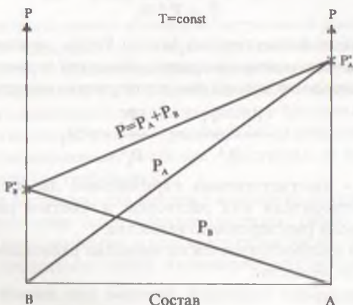
Рис. 9.1. Зависимость парциальных давлений насыщенных паров P_A , P_B и общего давления P = P_A + P_B от состава системы (выраженного в мольных долях), подчиняющейся закону Рауля.
