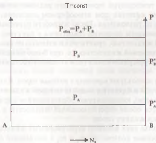
Рис. 10.5. Зависимость общего давления P_{\text{общ}} насыщенного пара, давлений P_A , P_B насыщенного пара над жидкими слоями компонентов А и В от состава системы при постоянной температуре.
