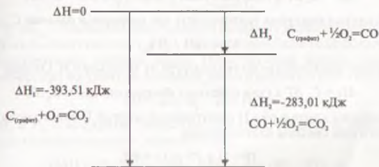
Рис. 2.1. Энтальпийная диаграмма для вычисления теплового эффекта реакции (3)
