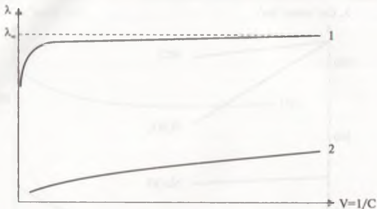
Рис. 15.4. Зависимость эквивалентной электропроводности \lambda растворов электролитов от разведения V = 1/C раствора: 1 – для сильных электролитов, 2 – для слабых электролитов.
