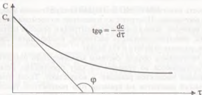
Рис. 18.2. К определению истинной скорости химической реакции по кинетической кривой. C — концентрация, \tau — время, C_0 — начальная концентрация реагента.
