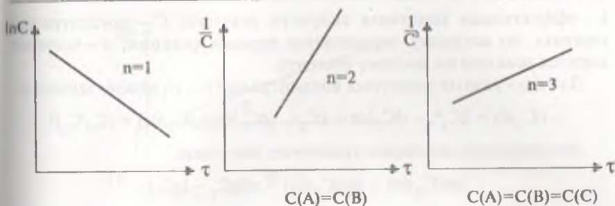
Рис. 18.6. Линейные зависимости функций концентрации ( \ln C , 1/C , 1/C^2 ) от времени \tau для реакций различного порядка n .
