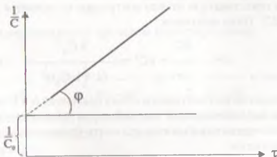
Рис. 18.4. Линейная зависимость обратной концентрации 1/C от времени \tau для реакции второго порядка при одинаковых начальных концентрациях реагентов
