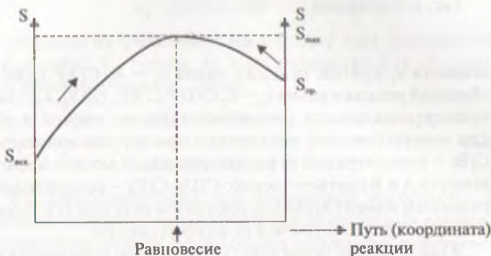
Рис. 5.3. Изменение энтропии S при протекании химической реакции в изолированной системе ( U = \text{const} , V = \text{const} ).
