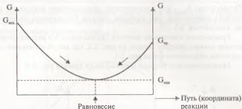
Рис. 5.1. Изменение энергии Гиббса G при протекании химической реакции в закрытой системе ( P = \text{const} , T = \text{const} ).
