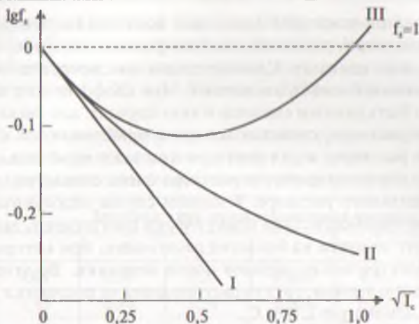
Рис. 13.3. Зависимость логарифма среднелионного коэффициента активности \lg \gamma_{\pm} от корня квадратного из ионной силы раствора \sqrt{I_c} . I — график функции (13.19) первого приближения теории Дебая и Хюккеля; II — график функции (13.23) второго приближения теории Дебая и Хюккеля; III — экспериментальная кривая.
