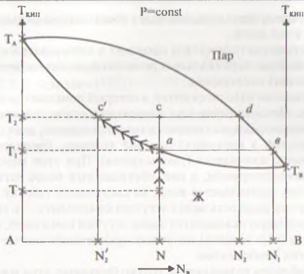
Рис. 9.9. Диаграмма кипения ( P = \text{const} ), иллюстрирующая сущность простой (однократной) перегонки. Обозначения — аналогичны обозначениям на рис. 9.8.
