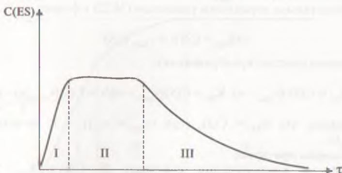
Рис. 24.2. Кинетическая кривая субстрат-ферментного комплекса ES; C(ES) — концентрация ES; \tau — время
