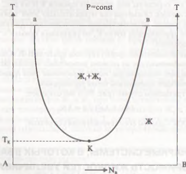
Рис. 10.2. Зависимость взаимной растворимости двух ограниченно смешивающихся жидкостей А и В от температуры T (при P = \text{const} ) с нижней критической температурой растворения. Обозначения — аналогичны обозначениям на рис. 10.1.
