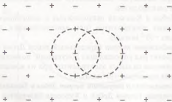
Рис. 13.2. Идеально упорядоченное распределение ионов в растворе. Пунктиром показано наличие ионной атмосферы .
