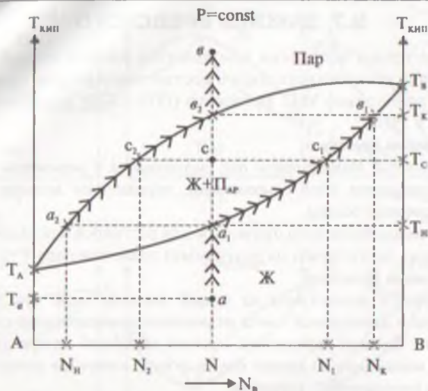
Рис. 9.8. Диаграмма кипения ( P = \text{const} ) бинарной смеси двух летучих жидкостей, неограниченно растворяющихся друг в друге.
