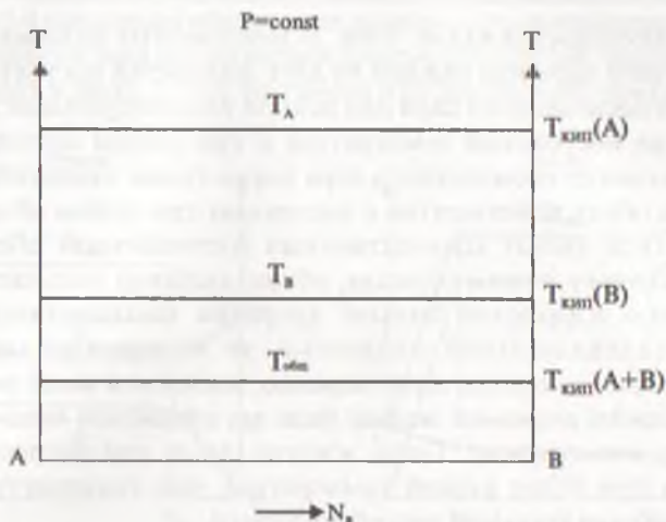
Рис. 10.6. Диаграмма кипения ( P = \text{const} ) смеси двух взаимно практически нерастворимых жидкостей А и В. T_{\text{кип}}(A) , T_{\text{кип}}(B) , T_{\text{кип}}(\text{смеси } A + B) — соответственно температура кипения чистых жидкостей А, В и смеси А + В.
