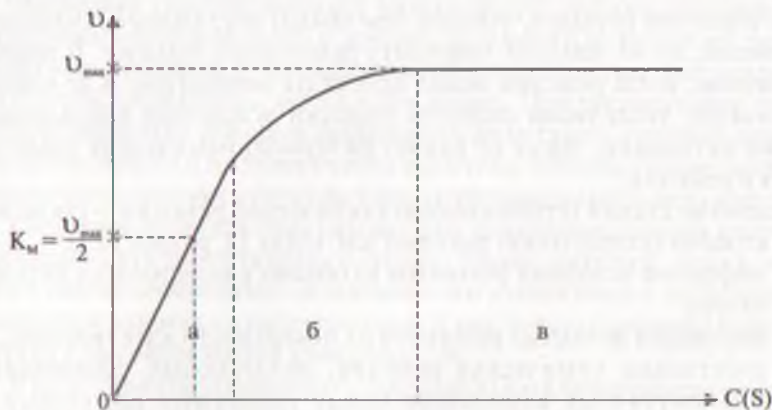
Рис. 24.3. Зависимость стационарной скорости v ферментативной реакции от концентрации субстрата C(S) . а — линейная область роста v , реакция — первого порядка; б — промежуточная область, порядок реакции изменяется от первого до нулевого; в — область насыщения, реакция — нулевого порядка. v_{\max} — максимальная скорость ферментативной реакции.
