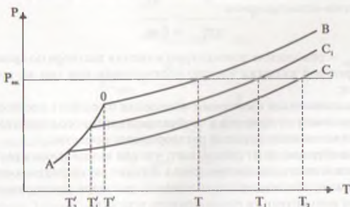
Рис. 12.1. Зависимость давления P насыщенного пара над разбавленным раствором нелетучего вещества от температуры T над твердой (АО) и жидкой ( B, C_1, C_2 ) фазами. P_{нн} — внешнее давление.
