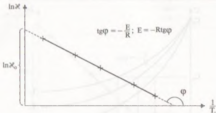
Рис. 19.4. График линейной зависимости логарифма коэффициента трансформации \ln k от обратной температуры 1/T . Крестиком обозначены величины, найденные опытным путем по кинетическим кривым.
