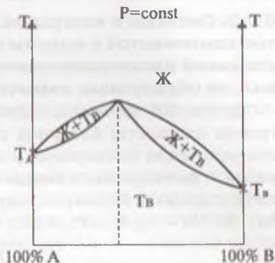
Рис 8.5. Диаграмма состояния (плавкости) двухкомпонентной системы изоморфно кристаллизующихся компонентов А и В с максимумом температуры плавления.
