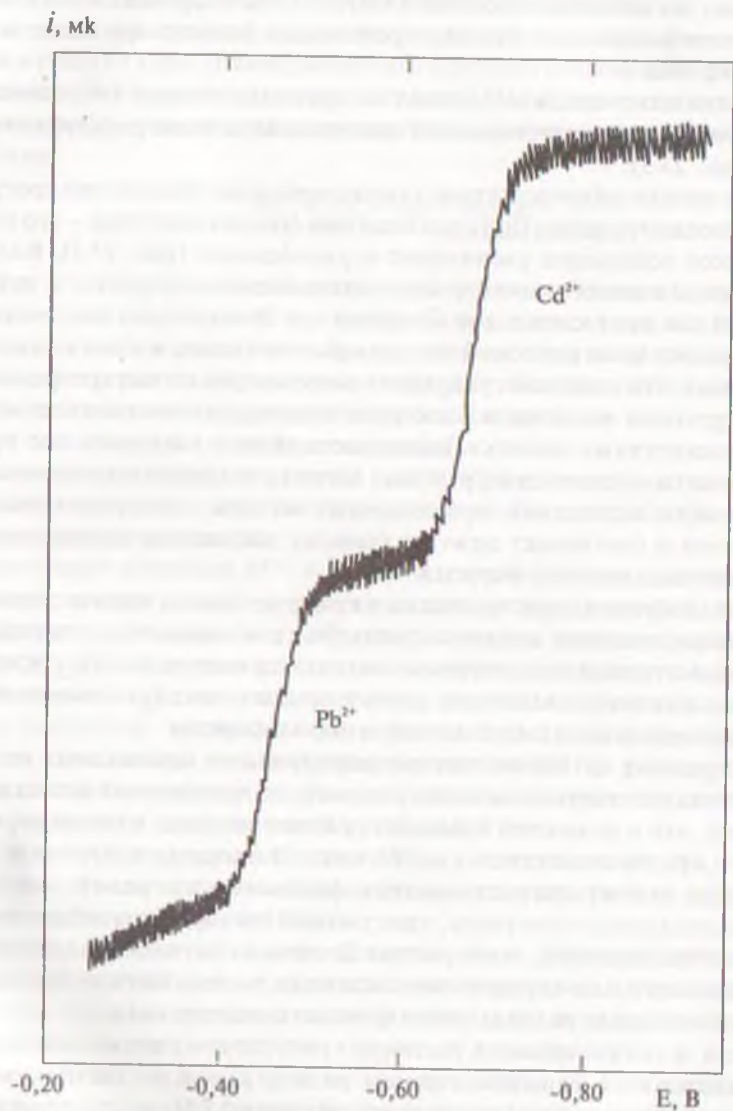
Рис. 23.4. Полярограмма раствора, содержащего катионы кадмия и свинца; i — ток, E — приложенный потенциал относительно потенциала насыщенного каломельного электрода.
