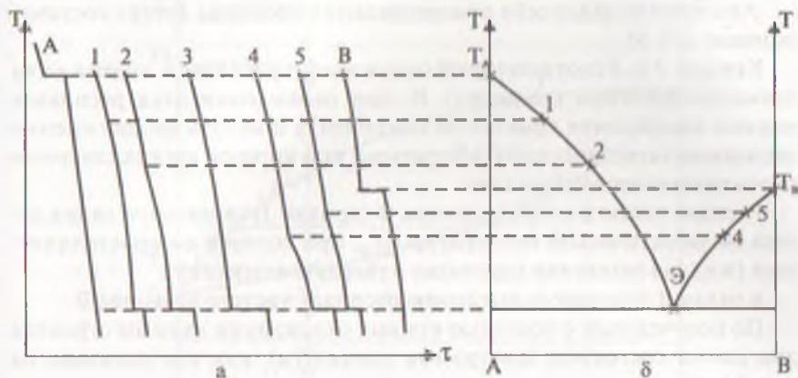
Рис. 8.2. Кривые охлаждения (a) и диаграмма плавкости (b) двухкомпонентной системы. T – температура, \tau – время.
