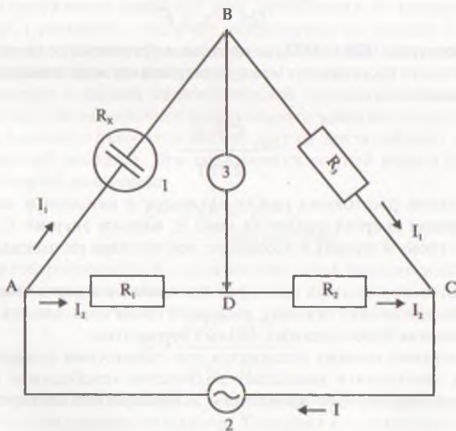
Рис. 15.6. Принципиальная схема для определения электрического сопротивления R_x раствора: 1 — электрохимическая ячейка с двумя электродами; 2 — источник переменного тока; 3 — нуль-прибор (индикатор); R_x , R_1 , R_2 , R_3 — сопротивления; I_1 , I_2 , I — ток.
