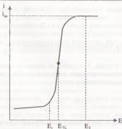
Рис. 23.1. Общий вид поляризационной (вольтамперной) кривой, характеризующей зависимость плотности тока i от потенциала электрода E . i_{\text{пр}} — предельный ток; E_1 — потенциал разряда (потенциал выделения); E_{1/2} — потенциал полуволны; E_2 — потенциал, соответствующий предельному току.
