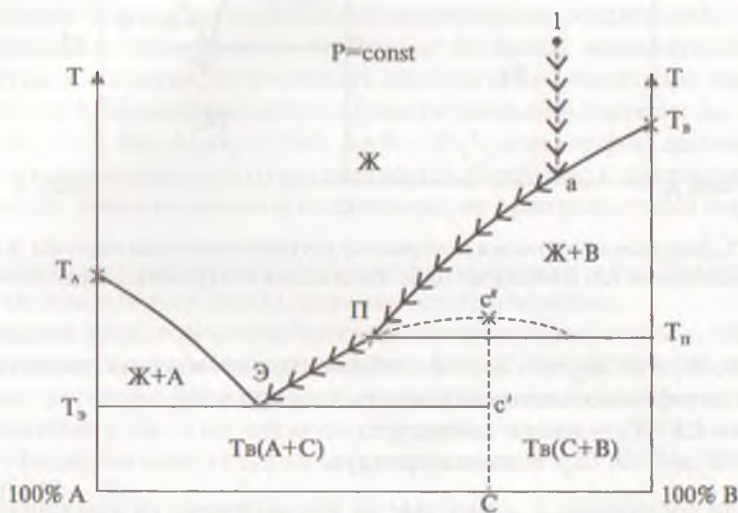
Рис. 8.8. Диаграмма состояния (плавкости) двухкомпонентной системы, в которой компоненты А и В образуют неустойчивое (плавящееся инконгруэнтно) соединение С. Пунктиром обозначен скрытый максимум, отвечающий температуре плавления чистого вещества С.
