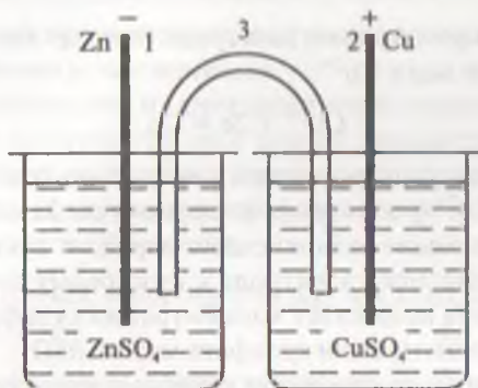
Рис. 17.2. Схема медноцинкового элемента Даниэля (Даниэля-Якоби): 1 — цинковая пластинка; 2 — медная пластинка; 3 — солевой мостик
