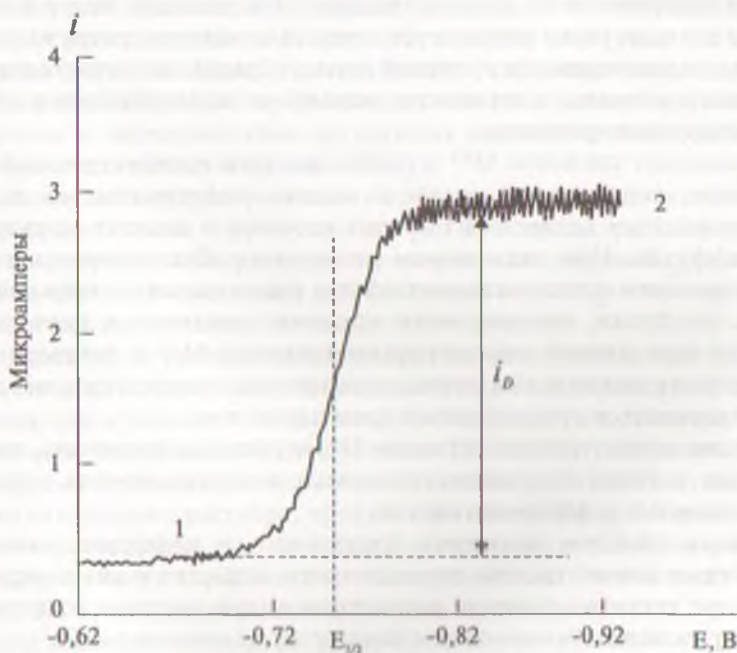
Рис. 23.3. Полярграмма водного щелочного 0,0005 моль/л раствора нитрата свинца при 25 °С ( i — ток, E — потенциал):
