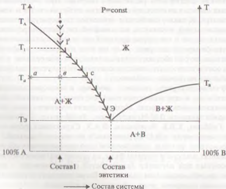
Рис. 8.1. Диаграмма состояния (плавкости) двухкомпонентной системы неизоморфно кристаллизующихся веществ с простой эвтектикой (не образующих химических соединений).
