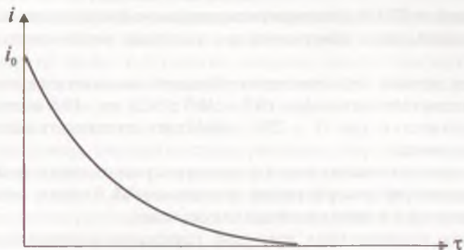
Рис. 23.6. Изменение тока i со временем \tau в прямой потенциостатической кулонометрии.
