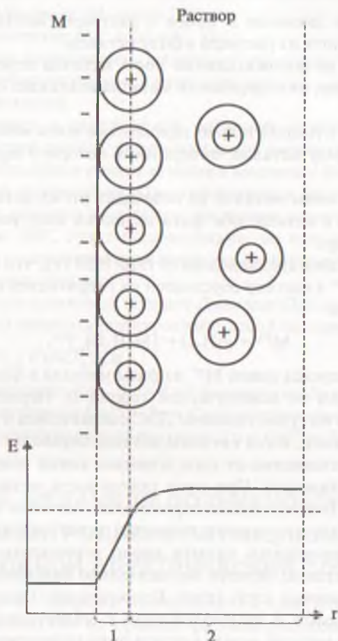
Рис. 16.1. Схематическое изображение двойного электрического слоя Гельмгольца – Гуи: 1 – плотный ДЭС; 2 – диффузный ДЭС; E – потенциал, g – расстояние от поверхности металла.
