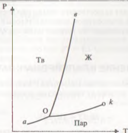
Рис. 7.3. Диаграмма состояния диоксида углерода \text{CO}_2 в координатах T , P (в закрытой системе).
