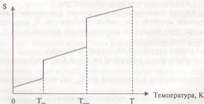
Рис. 3.2. Увеличение энтропии при нагревании вещества от T = 0 К до T .
