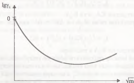
Рис. 13.1. Зависимость среднеионного коэффициента активности \gamma_{\pm} сильного электролита от его моляльности m в водном растворе.
