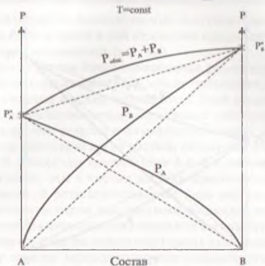
Рис. 9.2. Положительные отклонения от закона Рауля. Пунктирные линии соответствуют закону Рауля, сплошные — отвечают упругости пара в данной реальной системе. P_A^o , P_B^o — упругость насыщенного пара над чистыми компонентами А и В; P_A и P_B — парциальные упругости насыщенных паров компонентов А и В над раствором.
