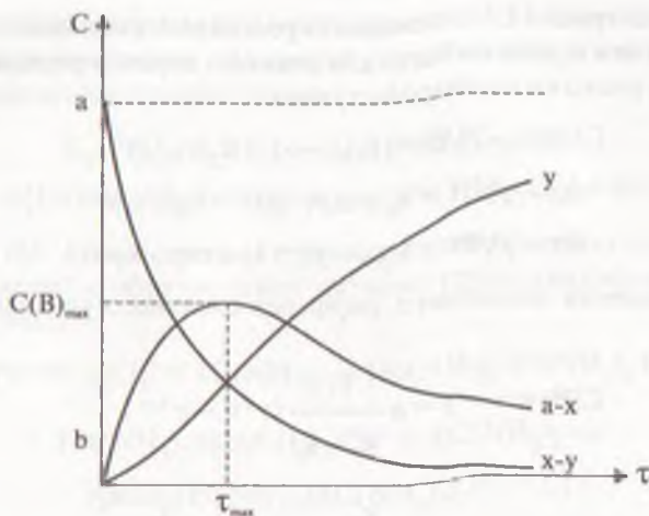
Рис. 18.9. Кинетические кривые для последовательных реакций первого порядка A \rightarrow B \rightarrow D . C – концентрация реагентов; \tau – время; a-x – концентрация реагента A ; x-y – концентрация промежуточного соединения B ; y – концентрация конечного продукта D ; \tau_{\max} – время максимального накопления промежуточного соединения при его максимальной концентрации C(B)_{\max} .
