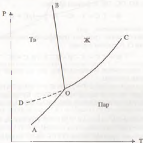
Рис. 7.1. Диаграмма состояния воды при давлениях P < 2,0266 \cdot 10^8 Па (в закрытой системе).
