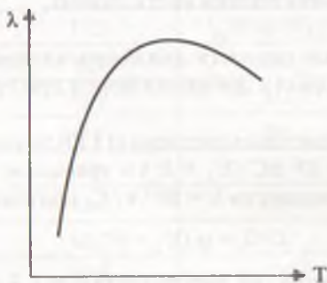
Рис. 15.5. Влияние температуры T на эквивалентную электропроводность \lambda слабого электролита.
