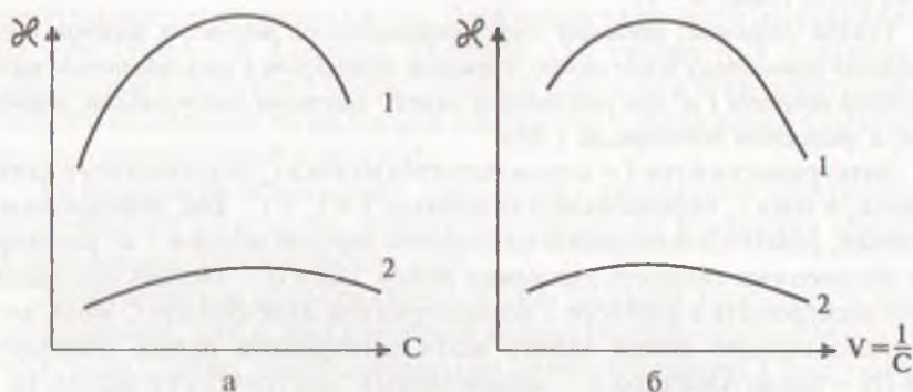
Рис.15.1. Общий вид зависимости удельной электропроводности \kappa растворов электролитов от концентрации C (а) и разведения V = 1/C (б) при постоянной температуре. 1 — для сильных электролитов, 2 — для слабых электролитов.
