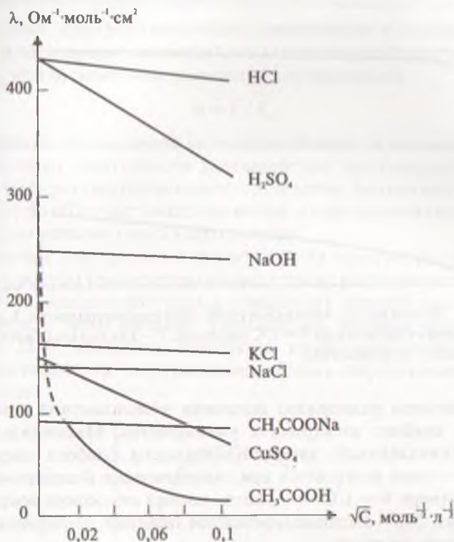
Рис. 15.3. Зависимость эквивалентной электропроводности \lambda растворов электролитов от корня квадратного C^{1/2} из молярной концентрации эквивалента раствора.
