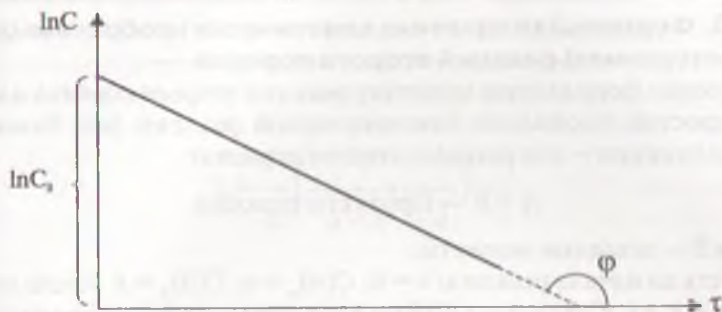
Рис. 18.3. Линейная зависимость \ln C от \tau для реакций первого порядка.
