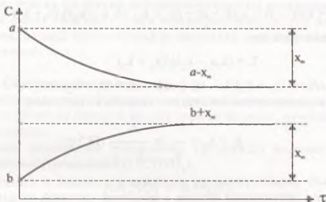
Рис. 18.8. Кинетические кривые для обратимой реакции A = B . C — концентрация реагентов; \tau — время; a, b — начальные концентрации реагентов A и B соответственно; x_\infty — изменение концентраций A и B от начала реакции до состояния равновесия.
