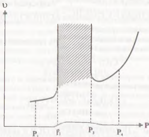
Рис. 21.2. Влияние давления P на скорость v разветвленной цепной реакции в газовой фазе:
