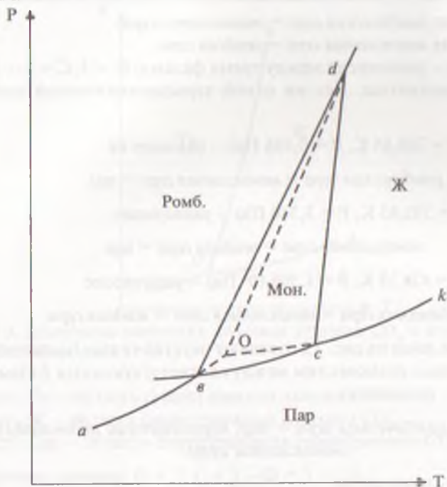
Рис. 7.2. Диаграмма состояния серы в координатах T , P (в закрытой системе).
