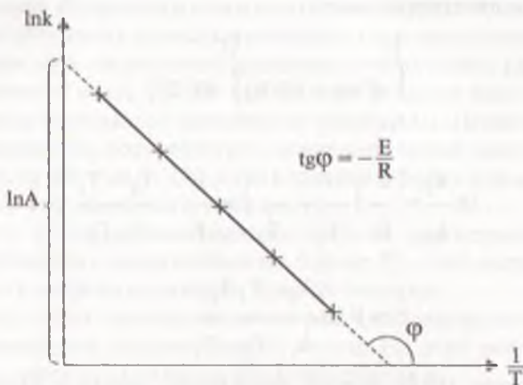
Рис. 19.2. График зависимости логарифма константы скорости реакции \ln k от обратной температуры 1/T . Крестиками обозначены опытные значения \ln k при разных 1/T
