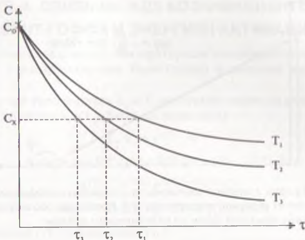
Рис. 19.3. Кинетические кривые при разных температурах T_1 < T_2 < T_3 . C — концентрация реагентов; C_0 — начальная концентрация реагентов; C_x — некоторая концентрация реагентов, соответствующая одинаковой степени их превращения в продуктах реакции.
