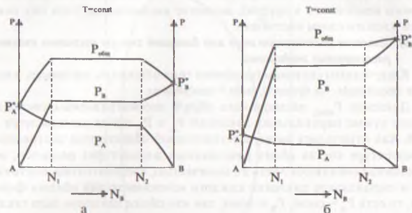
Рис. 10.4. Зависимость равновесного давления насыщенного пара над бинарной смесью жидкостей, ограниченно взаимно растворимых, от состава смеси при постоянной температуре T = \text{const} : а — случай P_{\text{общ}} > P_A^0, P_{\text{общ}} > P_B^0 ; б — случай P_A^0 < P_{\text{общ}} < P_B^0 .
