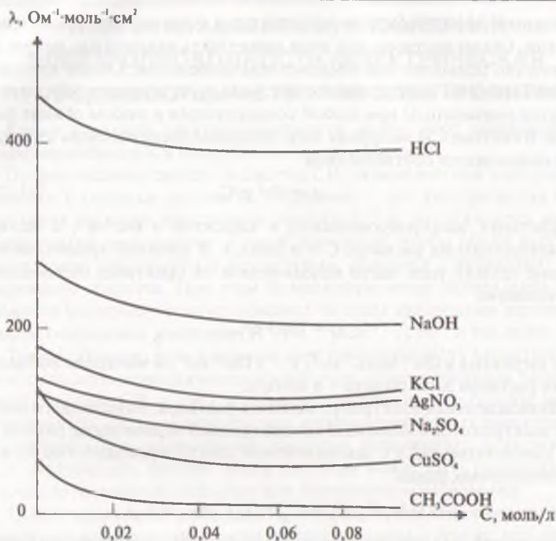
Рис. 15.2. Зависимость эквивалентной электропроводности \lambda водных растворов электролитов от их концентрации C (молярной концентрации эквивалента).
