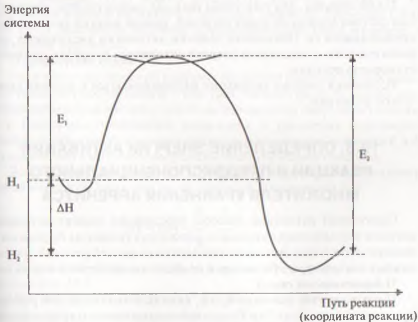
Рис. 19.1. Изменение энергии реагирующей системы по ходу реакции. E_1 — энергия активации прямой реакции; E_2 — энергия активации обратной реакции; \Delta H = H_2 - H_1 — тепловой эффект реакции при постоянном давлении (разность энтальпий H_2 продуктов реакции и энтальпий H_1 исходных реагентов). Путь реакции — переход от исходных реагентов к продуктам реакции
