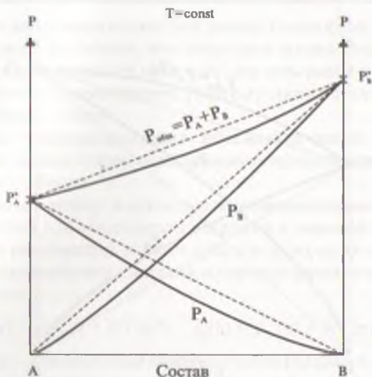
Рис. 9.3. Отрицательные отклонения от закона Рауля. Пунктирные линии отвечают закону Рауля, сплошные — упругости пара в данной реальной системе. P_A^\circ, P_B^\circ — упругость насыщенного пара над чистым компонентом А и В; P_A, P_B — упругость насыщенного пара компонентов А и В над раствором.
