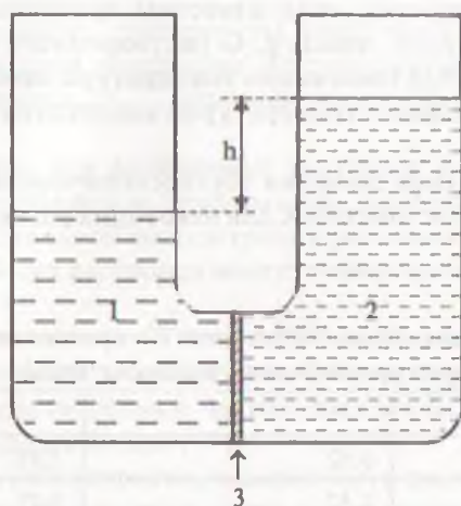
Рис. 12.2. Схема возникновения осмотического давления: 1 — растворитель, 2 — раствор, 3 — полупроницаемая перегородка (мембрана).
