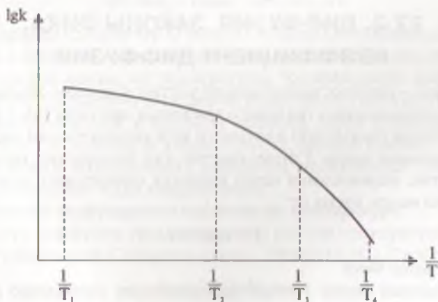
Рис. 22.1. Зависимость логарифма константы скорости \lg k гетерогенной химической реакции от обратной температуры 1/T . Области от 1/T_1 до 1/T_2 , от 1/T_2 до 1/T_3 и от 1/T_3 до 1/T_4 — соответственно диффузионная, переходная и кинетическая области процесса.
