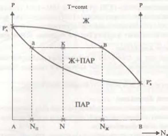
Рис. 9.6. Диаграмма зависимости давления насыщенного пара от состава бинарной системы при постоянной температуре.
