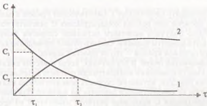
Рис. 18.1. Кинетические кривые ( C — концентрация, \tau — время): 1 — для исходного реагента, 2 — для продукта реакции.
