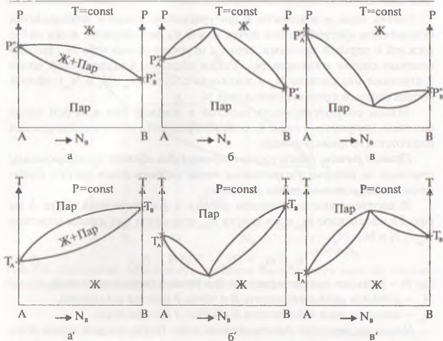
Рис. 9.7. Основные типы диаграмм P = f(N) (а, б, в) и T_{\text{кип.}} = f(N) (а', б', в') бинарных систем полностью взаимно растворимых жидкостей.
