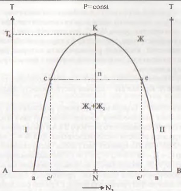
Рис. 10.1. Зависимость взаимной растворимости двух ограниченно смешивающихся жидкостей А и В от температуры T при постоянном давлении P = \text{const} с верхней критической температурой растворения ( N_B — мольная или массовая доля компонента В).
