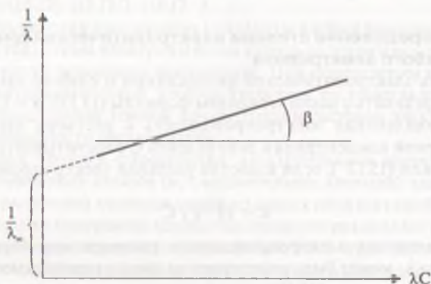
Рис. 15.7. Зависимость 1/\lambda от \lambda C ( \lambda — эквивалентная электропроводность раствора электролита с молярной концентрацией эквивалента C ).
