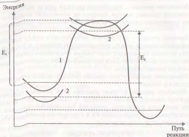
Рис. 21.1. Иллюстрация влияния сольватации на энергию активации реакции. E_1 — энергия активации реакции при отсутствии сольватации, E_2 — энергия активации реакции при сольватации исходных реагентов и активированного комплекса.
