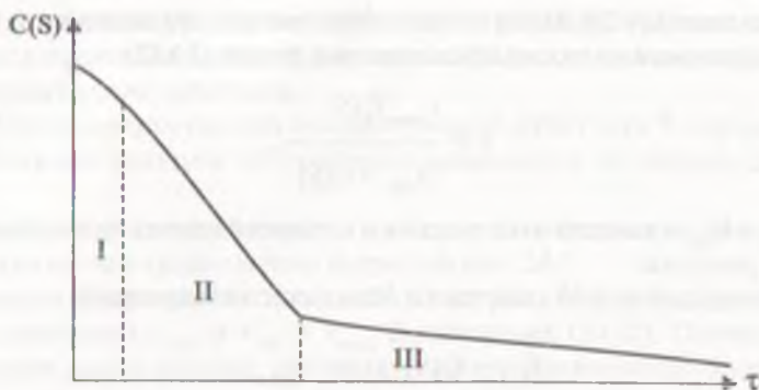
Рис. 24.1. Кинетическая кривая субстрата S; C(S) — концентрация субстрата S; \tau — время
