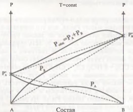
Рис. 9.4. Система, в которой наблюдаются положительные и отрицательные отклонения от закона Рауля. Пунктирные линии отвечают закону Рауля, сплошные — реальной упругости пара в системе. P_A^\circ, P_B^\circ — упругость насыщенного пара над чистыми компонентами А и В; P_A, P_B — парциальные упругости насыщенного пара компонентов А и В над раствором.
