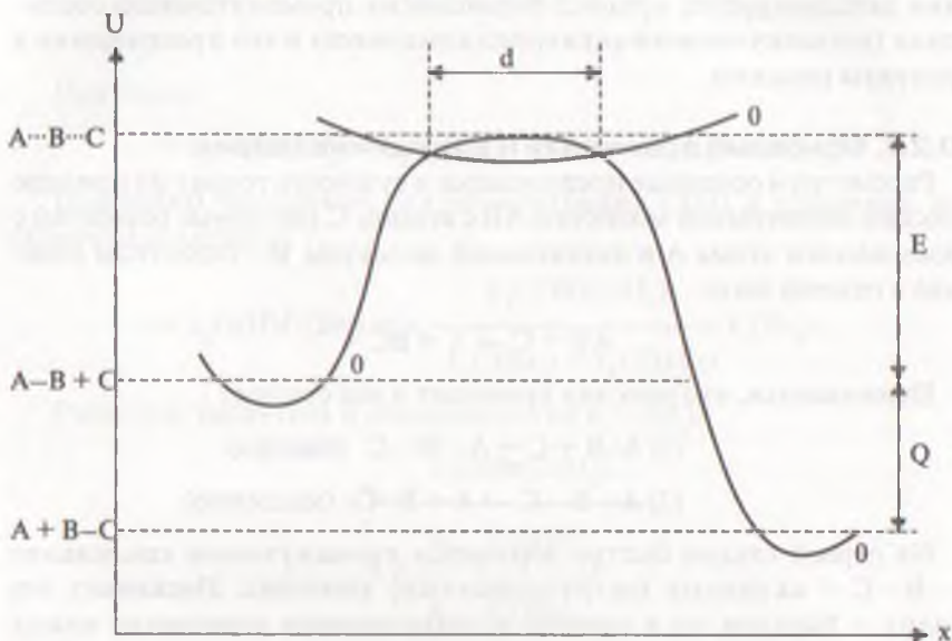
Рис. 20.1. Энергетический профиль реакции A-B + C \rightleftharpoons A-B \cdots C \rightarrow A + B-C . U — потенциальная энергия системы; x — координата реакции (путь реакции); E — энергия активации реакции; \delta — ширина максимума потенциального барьера. Нулями обозначены нулевые энергетические уровни.
