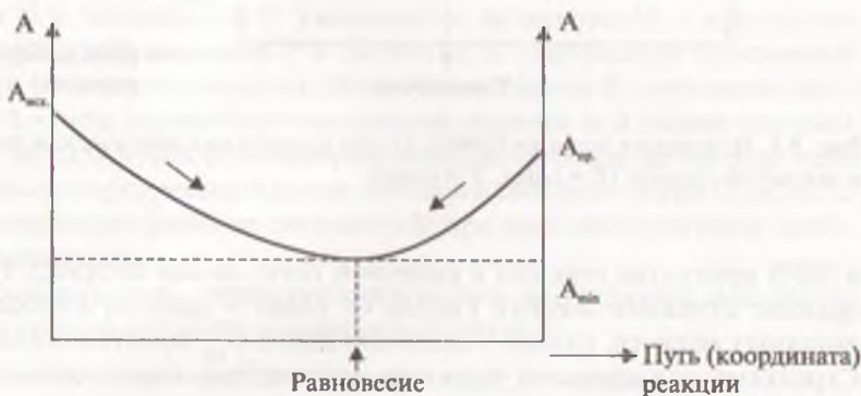
Рис. 5.2. Изменение энергии Гельмгольца A при протекании химической реакции в закрытой системе ( V = \text{const} , T = \text{const} ).
