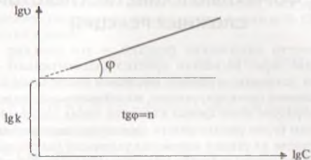
Рис. 18.7. Линейная зависимость логарифма скорости реакции v от логарифма концентрации C реагента; n — частный порядок реакции по данному реагенту; k — эффективная константа скорости реакции.
