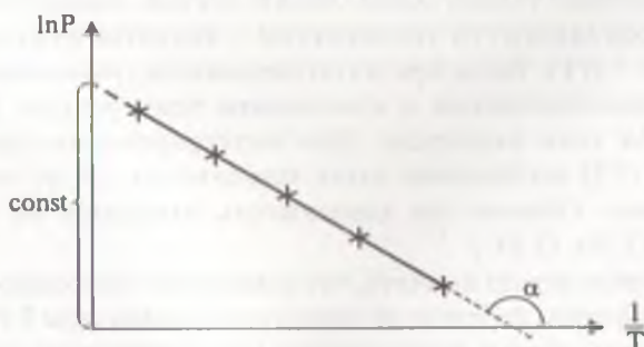
Рис. 7.4. Зависимость \ln P от 1/T при \Delta H_{\text{ср}} = \text{const} .
